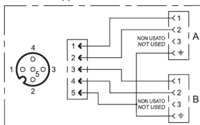
СХЕМА ПОДКЛЮЧЕНИЯ РАЗЪЕМА M12X1
