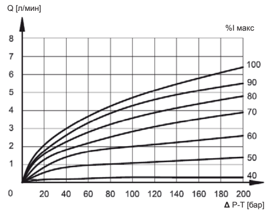
ТИП ЗОЛОТНИКА С01
