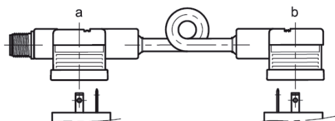
подключение разъема DUAL DIN 43650 тип разъема K12
